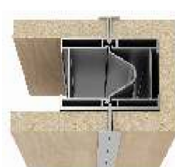
Spojení panelů
